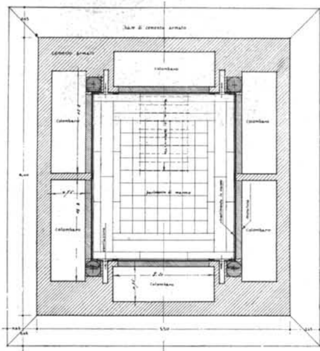
Pianta del sotterraneo (colombari)
