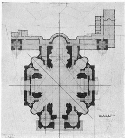
Sopra: IL BOZZETTO - In basso a sinistra: PLANIMETRIA GENERALE - A destra: PIANTE DELLA CHIESA.
